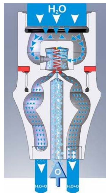
ABB. 2: SCHNITT VV7
